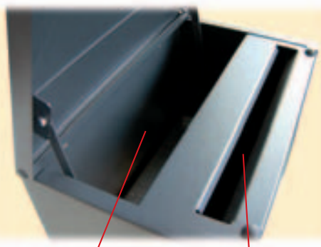
Medidas entrada paquetes: 276 x 85 mm.
